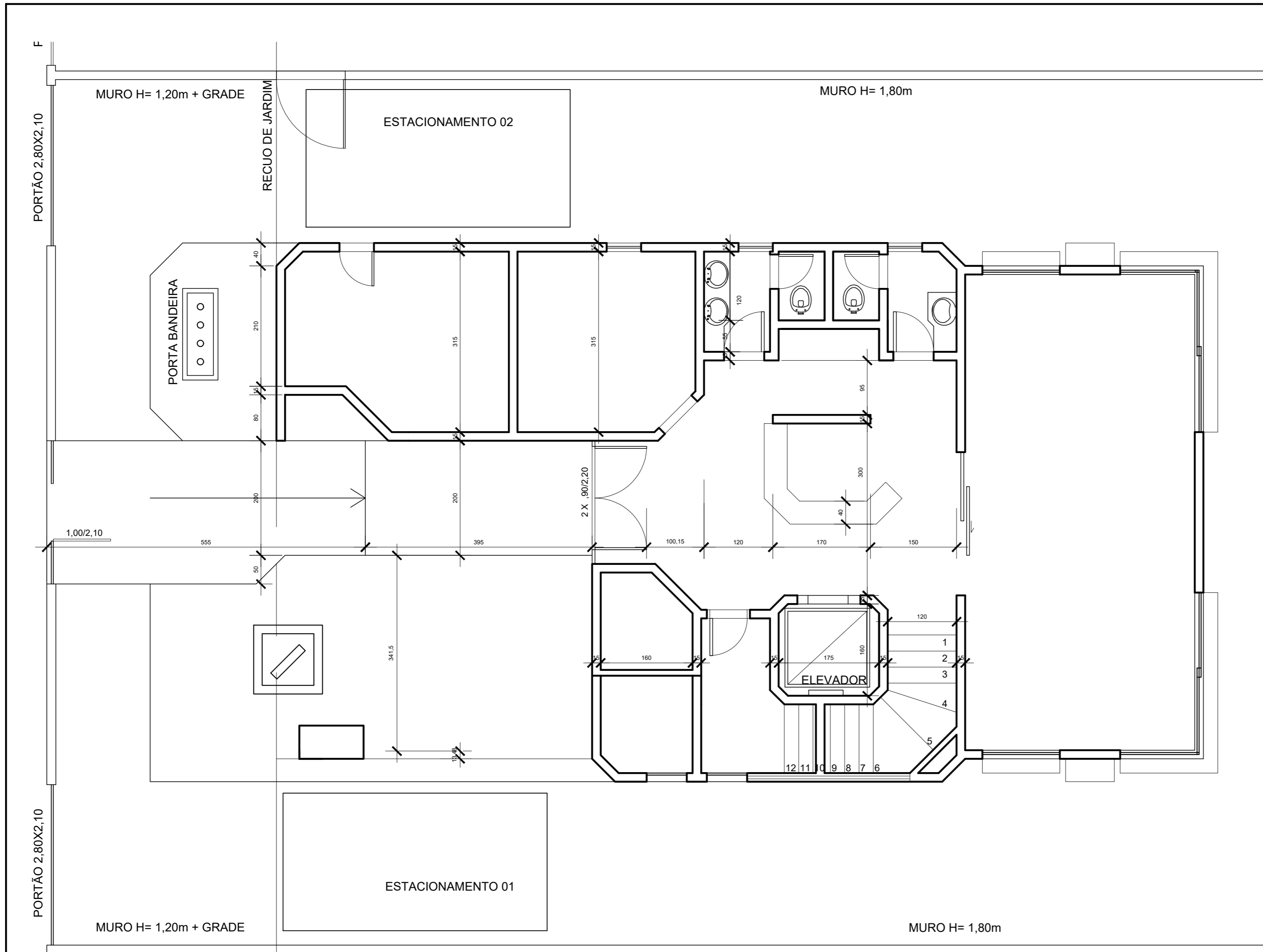
TERREO ATUAL ESCALA 1/50
