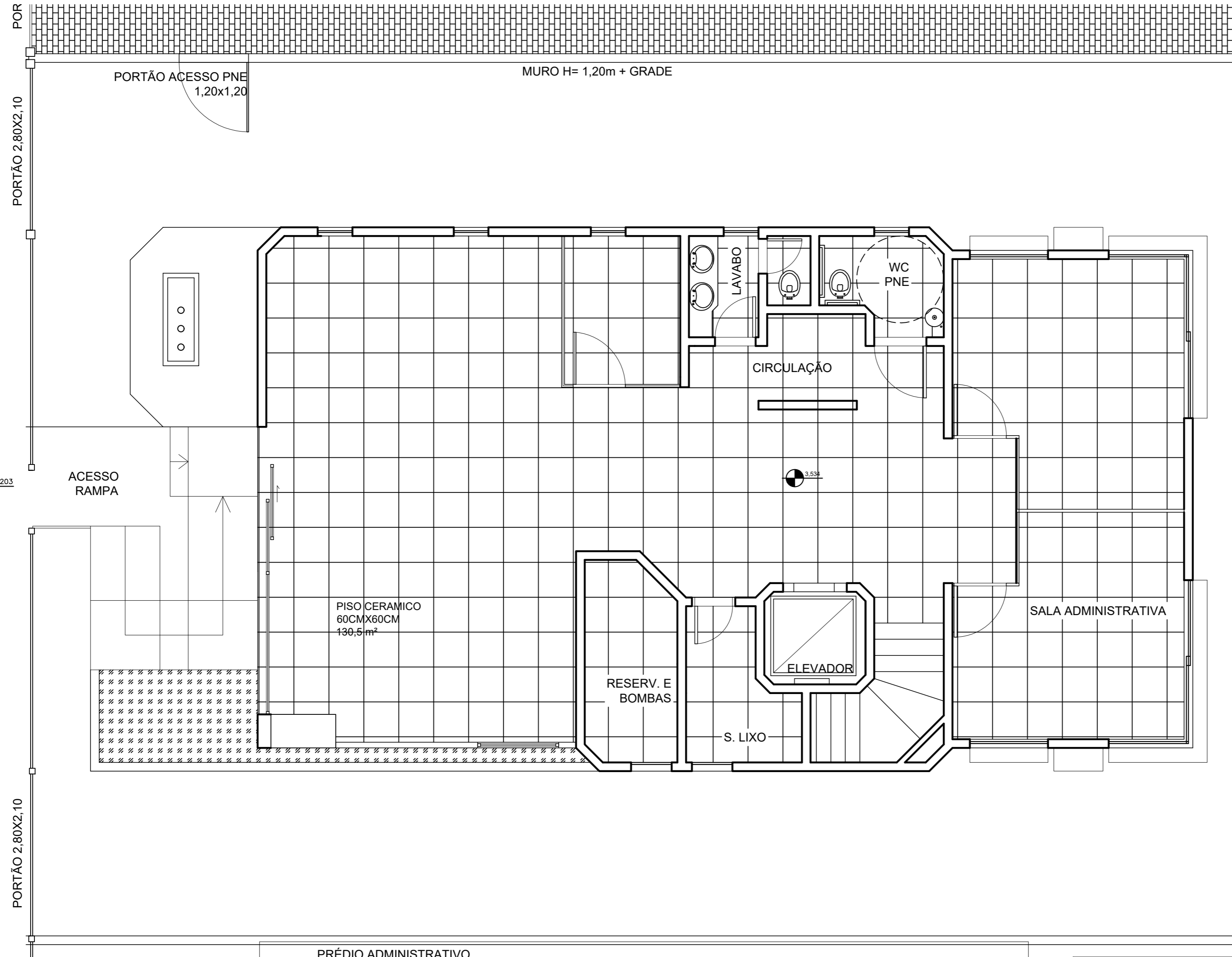
TERREO DETALHAMENTO PISO ESCALA 1/50
